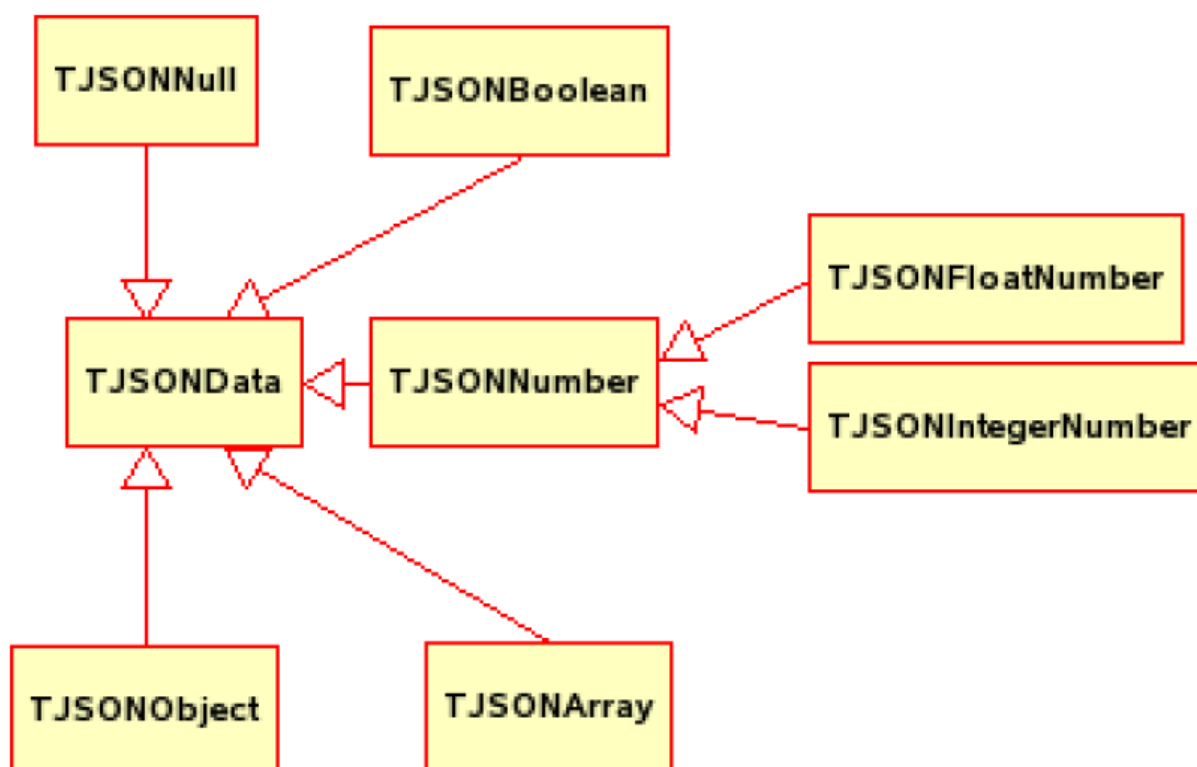
Рисунок 2: Структура данных JSON в fpjson
