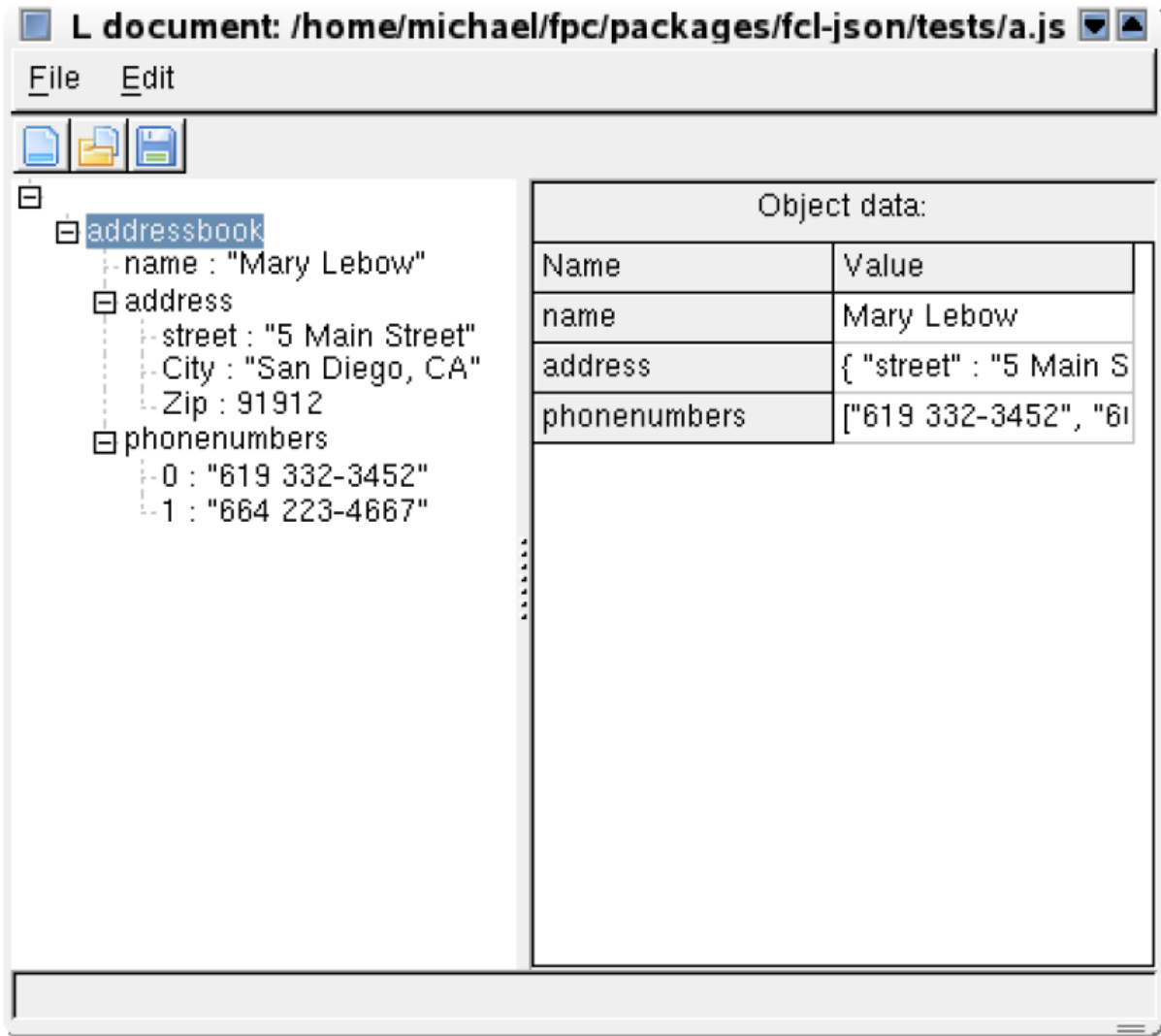
Рисунок 3: Приложение просмотра JSON
