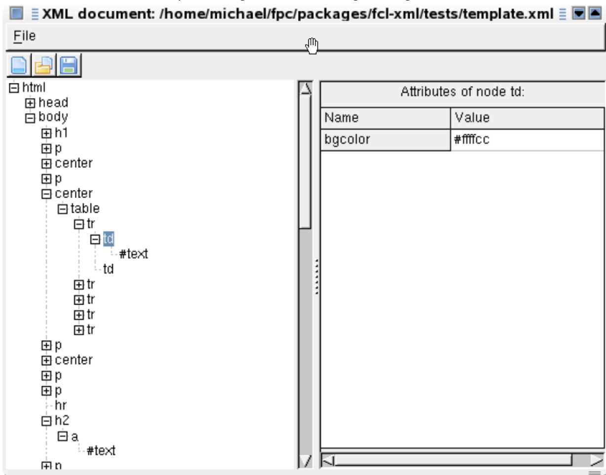
Рисунок 1: Приложение для просмотра XML
